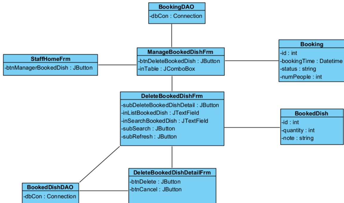
Sơ đồ lớp thiết kế
