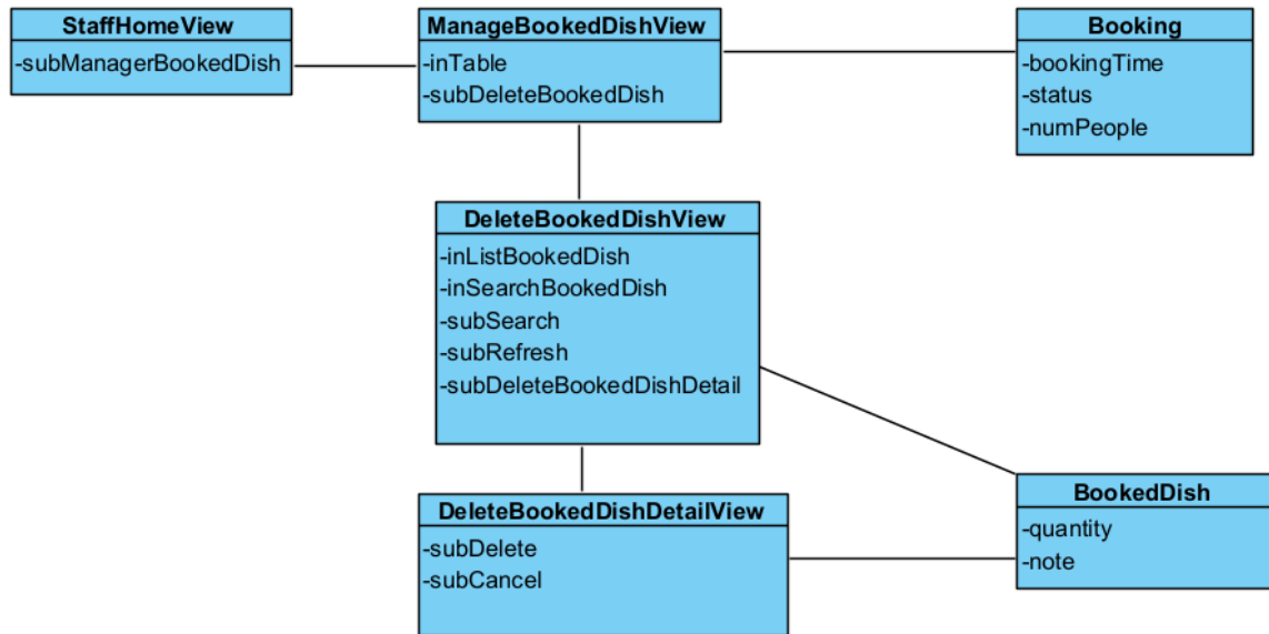
Sơ đồ lớp phân tích
